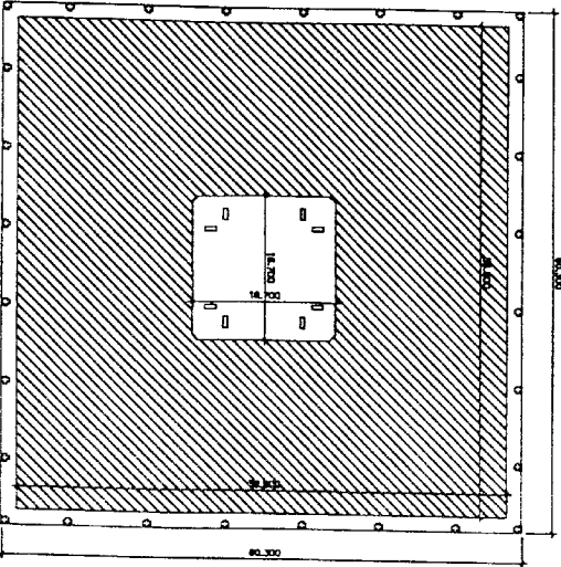
ΔΙΑΓΡΑΜΜΑ Α' ΟΡΟΦΟΥ ΚΑΤΑΣΤΑΣΗ ΠΡΟΤΥΠΟΥ ΚΑΙ ΔΙΑΣΤΑΣΕΙΣ ΚΑΤΑΣΤΑΣΗΣ ΚΑΤΑΣΤΑΣΗ ΠΡΟΤΥΠΟΥ ΚΑΙ ΔΙΑΣΤΑΣΕΙΣ ΚΑΤΑΣΤΑΣΗΣ ΚΑΤΑΣΤΑΣΗ ΠΡΟΤΥΠΟΥ ΚΑΙ ΔΙΑΣΤΑΣΕΙΣ ΚΑΤΑΣΤΑΣΗΣ
